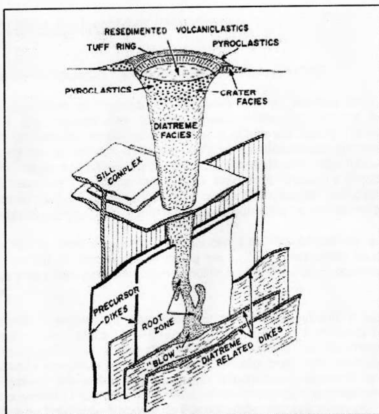
Figura 02 – Modelo clássico de "pipe" kimberlítico do tipo Sul-Africano, segundo Clement (1975), modificado por Mitchel (1986).
