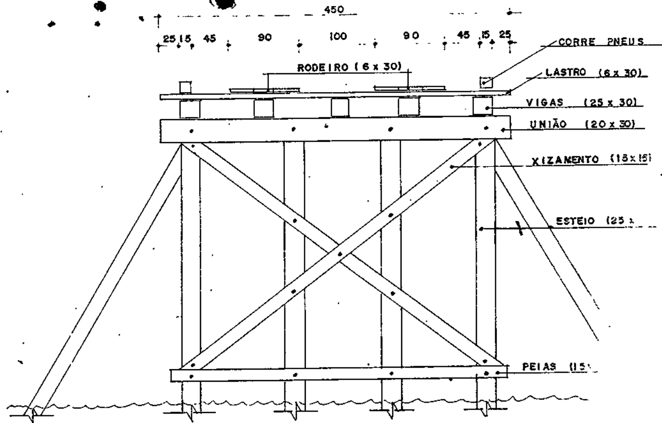
CORTE TRANSV. ESC: 1/50
