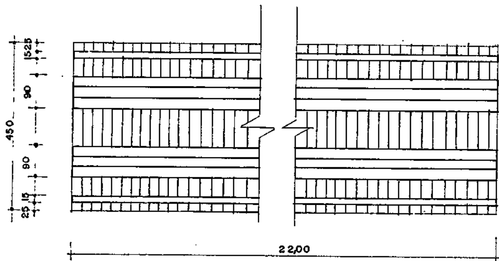
PLANTA ESC: 1/100
