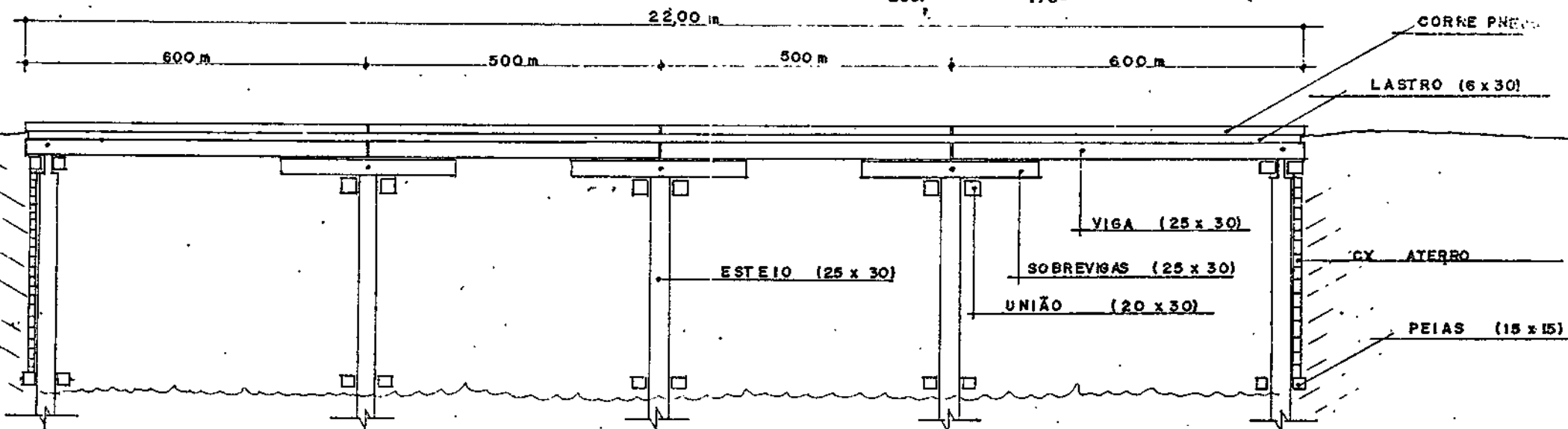
CORTE LONG
