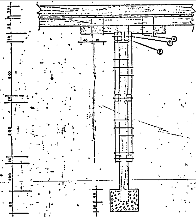
DETALHE DAS EMENDAS DOS ESTEIOS
