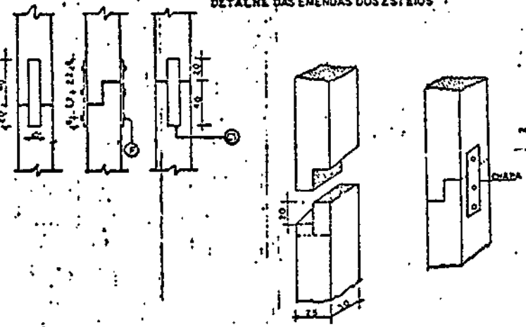
DETALHE DAS EMENDAS DOS ESTEIOS
