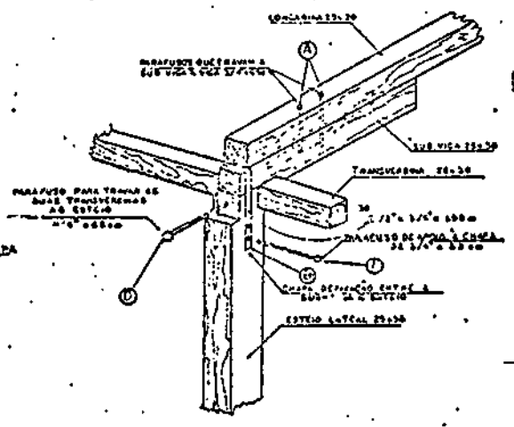
ESTEIO LATERAL DETALHE DO TRAVAMENTO ENTRE OS ESTEIOS, AS TRANSVERSINAS, SUB-VIGA E LONGARINAS.
