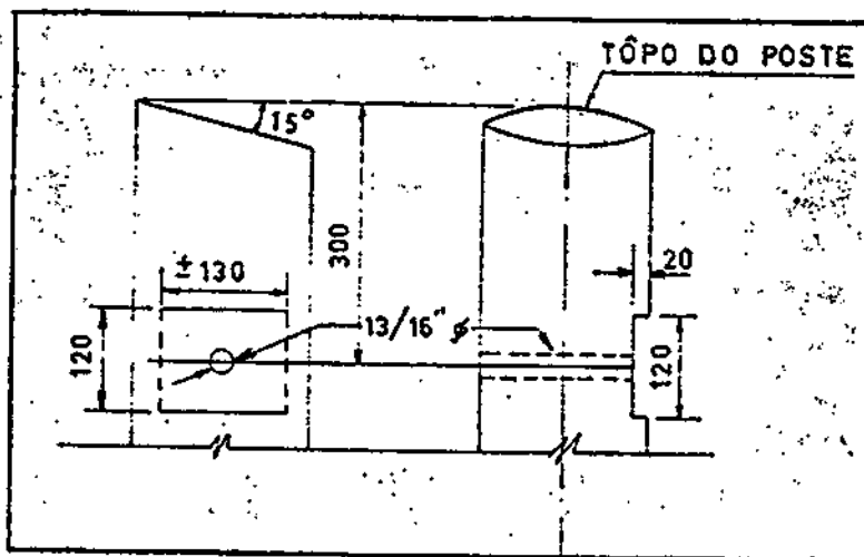
Fig.nº 2 - Tópo e encaixe nos postes de madeira
