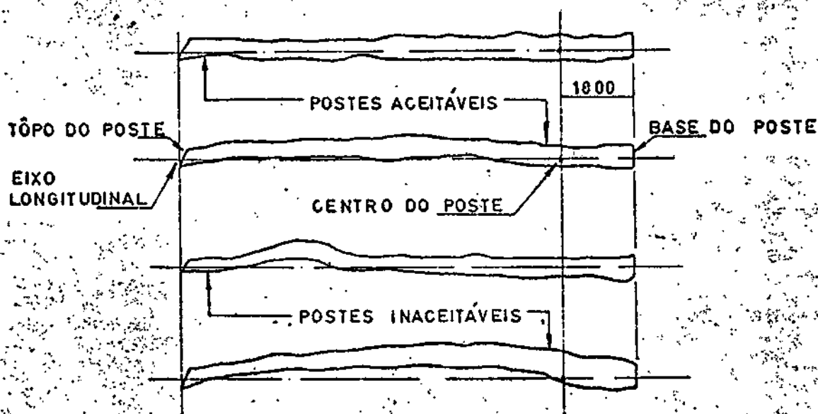
Fig.nº1 - Postes de madeira aceitáveis em relação ao eixo longitudinal.
